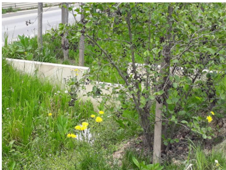
Figure 3 : Noue à redans le long d'une voirie – ARNOULD W.
