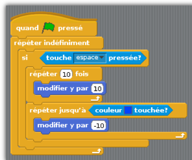
Un exemple de code avec Scratch
